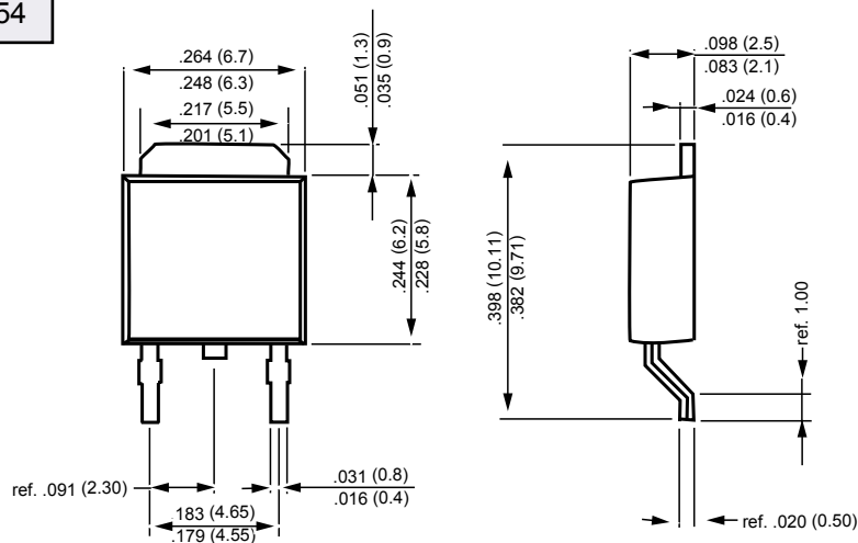
D-PAK
