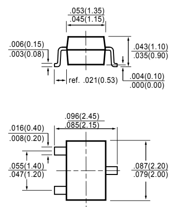
SOT-323
